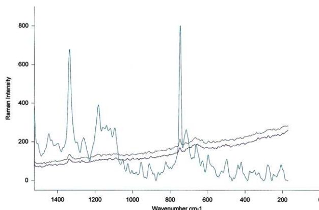
Ryc. 6. Widma ramanowskie tonera i pasty długopisowej.
