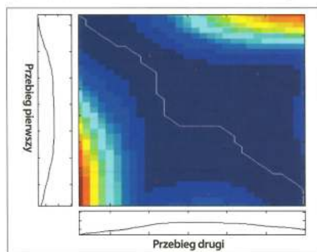
Ryc. 2. Macierz kosztów przejścia z optymalną ścieżką dopasowania DTW. Ciepłsze kolory oznaczają większy koszt przejścia niż kolory chłodniejsze
