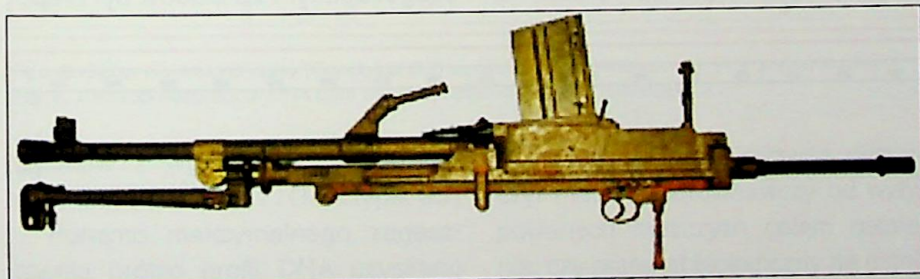
Ryc. 14. Przedmiotowy rkm BREN kal. 7,92 mm „Mauser” z magazynkiem pochodzącym od rkm-u ZB 26 Fig. 14. BREN cal. 7.92 mm „Mauser” with magazine originating from ZB 26 hand machine-gun
