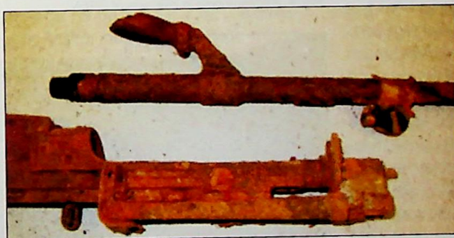
Ryc. 5. Rura gazowa z dwójnogiem oraz część lufy rkm-u BREN w stanie nadesłanym do badań
