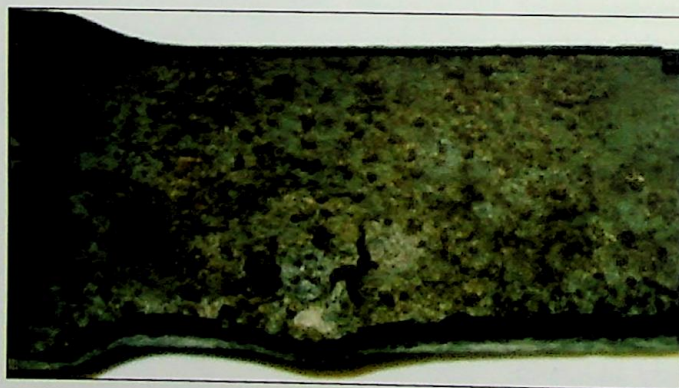
Ryc. 9. Otwór wylotowy w rurze gazowej badanego rkm-u BREN Fig. 9. Outlet hole in gas pipe of BREN
