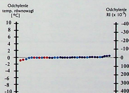
Ryc. 17. Brak efektów powierzchniowych dla pomiarów RI (brak anomalii) Fig. 17. Lack of surface effects for RI measurements (no anomalies)
