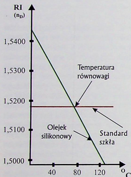
Ryc. 33. Zależność RI oleju silikonowego i szkła od temperatury Fig. 33. Dependence of RI of silicon oil and glass on temperature
