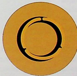
Ryc. 46. Nieprawidłowo wycentrowana kondensorowa przysłona pierścieniowa z pierścieniem fazowym obiektywu Fig. 46. Incorrectly centered condensing ring shutter with lenses phase ring
