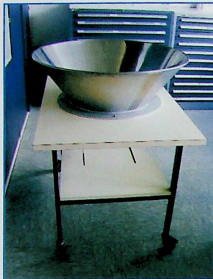
Ryc. 28. Stalowy lejek stosowany w BKA (Wiesbaden) do zbierania wytrzepin z odzieży Fig. 28. Steel funnel used in BKA (Wiesbaden) for collection of shaken off clothes particles
