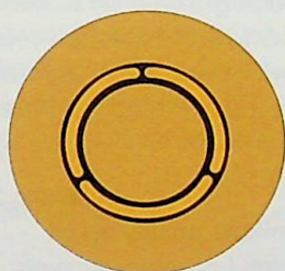
Ryc. 45. Prawidłowo wycentrowana kondensorowa przysłona pierścieniowa z pierścieniem fazowym obiektywu Fig. 45. Correctly centered condensing ring shutter with lenses phase ring
