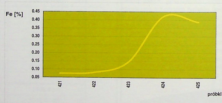
Ryc. 26. Zmiana zawartości Fe w czasie zmiany barwy tafli szkła float (pomiar powierzchni niefloat za pomocą spektrometru XRF ED X-lab 2000 firmy Spectro) Fig. 26. Change of Fe content in colour transition of float glass (non-float surface measurement by means of XRF ED X-lab 2000 [Spectro] spectrometer)
