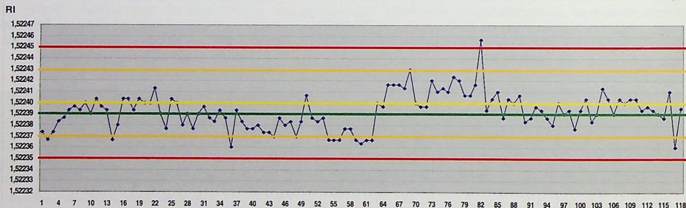
Ryc. 41. Wykres wyników pomiarów RI szkła wzorcowego od 23.04.2002 r. do 3.03.2004 r. opracowany na podstawie karty Shewarta Fig. 41. Results of RI measurements of glass standard (from 23-04-2002 to 03-03-2004) developed basing on Shewart's cart
