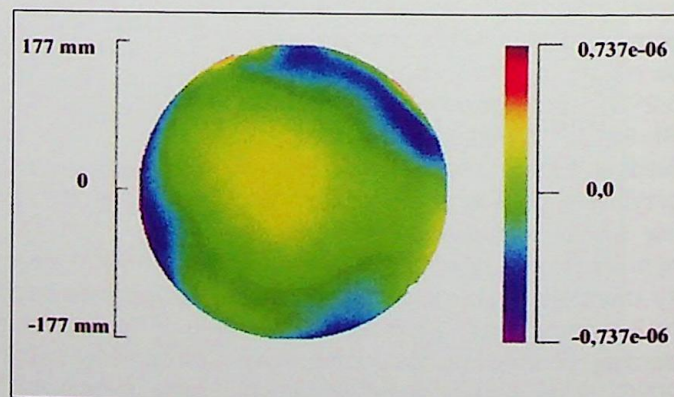
Ryc. 40. Homogeniczność wzorca BKA-5 Fig. 40. Homogeneity of BKA-5 standard
