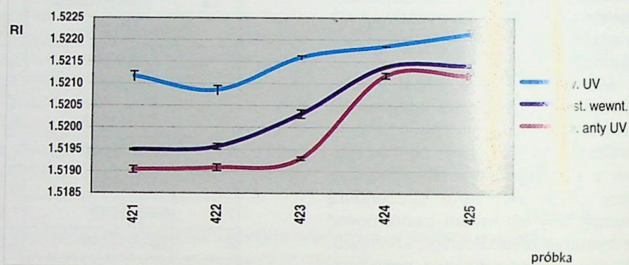
Ryc. 25. Zmiana RI poszczególnych warstw w czasie zmiany barwy tafli szkła float Fig. 25. Change of RI of specific layers in relation to change of float glass colour
