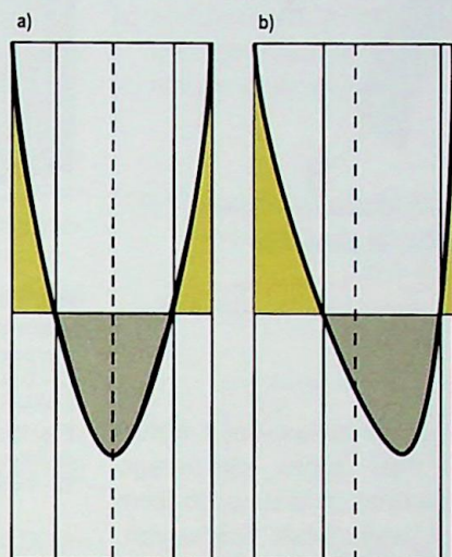
Ryc. 15. Schemat rozkładu sił wewnętrznych (naprężeń) w szkło: a) rozkład symetryczny, b) rozkład asymetryczny Fig. 15. Distribution of internal forces in glass: a) symmetrical distribution, b) asymmetrical distribution
