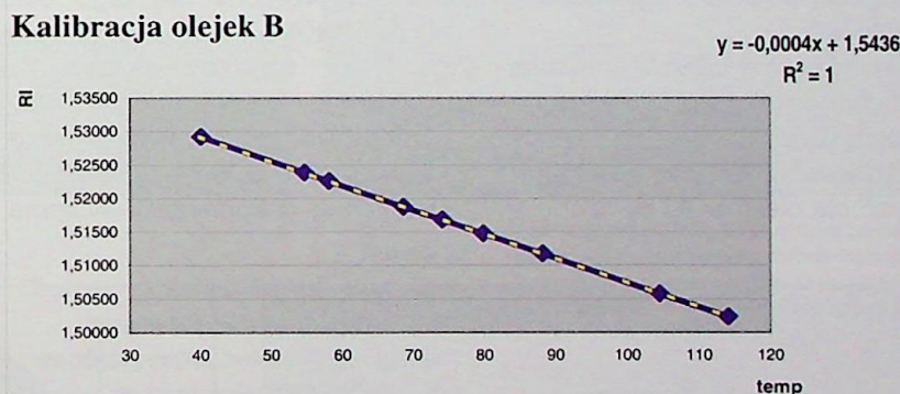
Ryc. 37. Krzywa kalibracyjna wzorców szkła w olejku B Fig. 37. Calibration curve for glass standard in oil B
