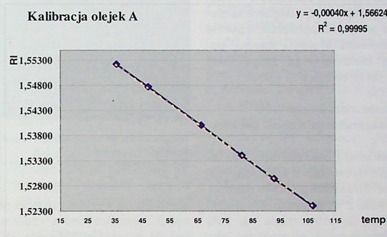
Ryc. 36. Krzywa kalibracyjna szkła wzorcowych w olejku A Fig. 36. Calibration curve for glass standard in oil A
