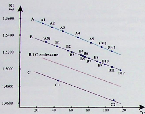
Ryc. 35. Zmiany RI z temperaturą dla olejków silikonowych typu A, B i C (światło sodowe – 589 nm) Fig. 35. RI changes with temperature for silicon oils A, B and C (sodium light – 589 nm)
