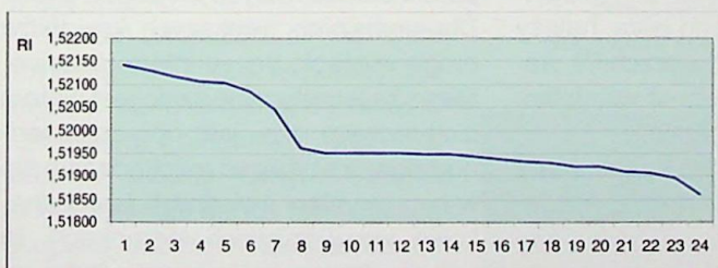
Ryc. 27. Graficzny obraz zmienności RI w szkła float od powierzchni UV do powierzchni anty-UV
